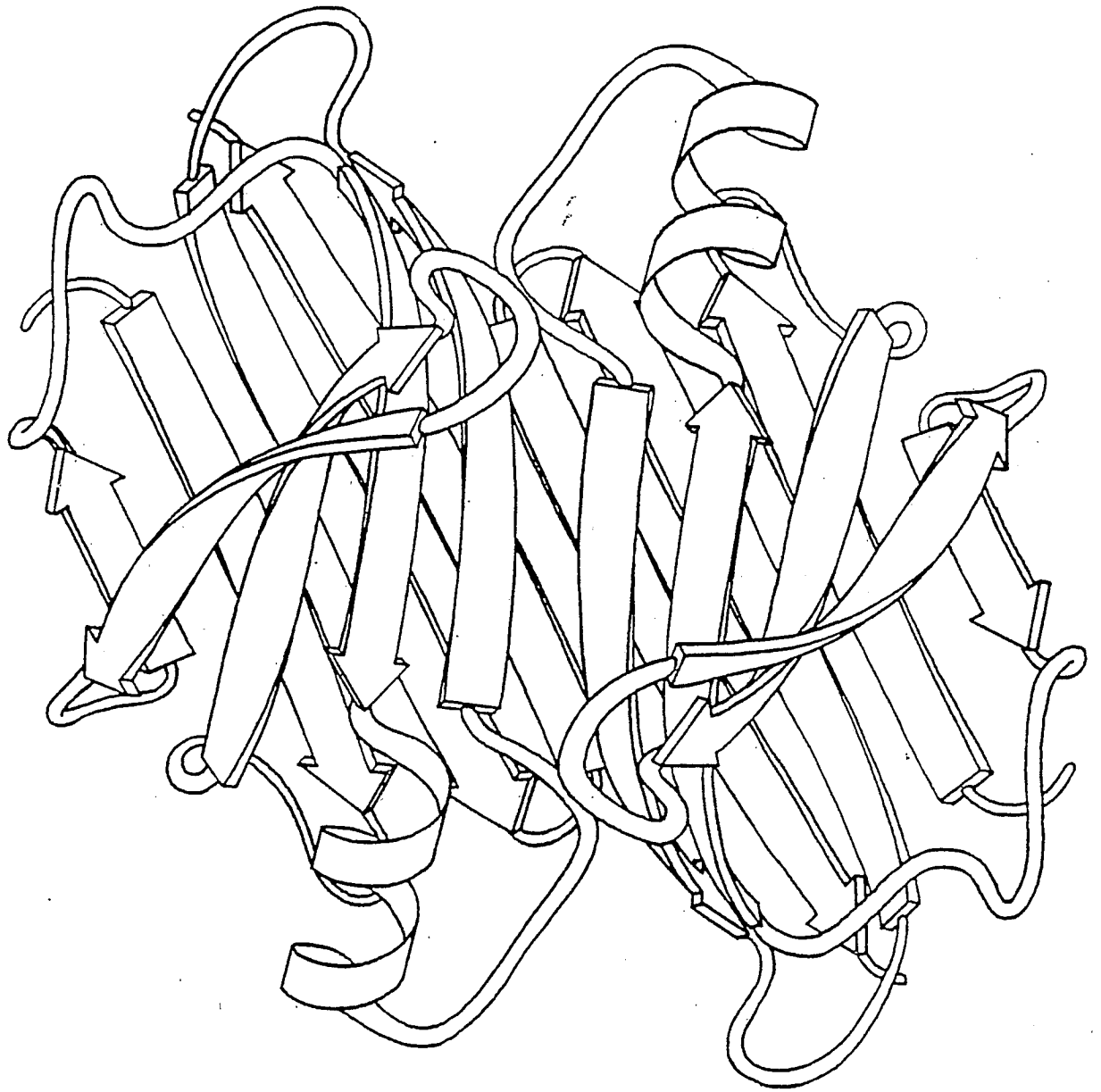
Prealbumin Dimer
