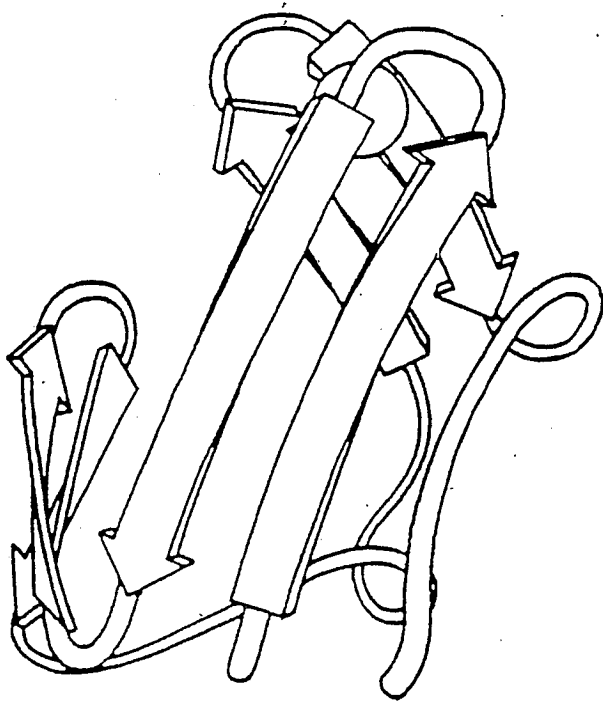
Rubredoxin
