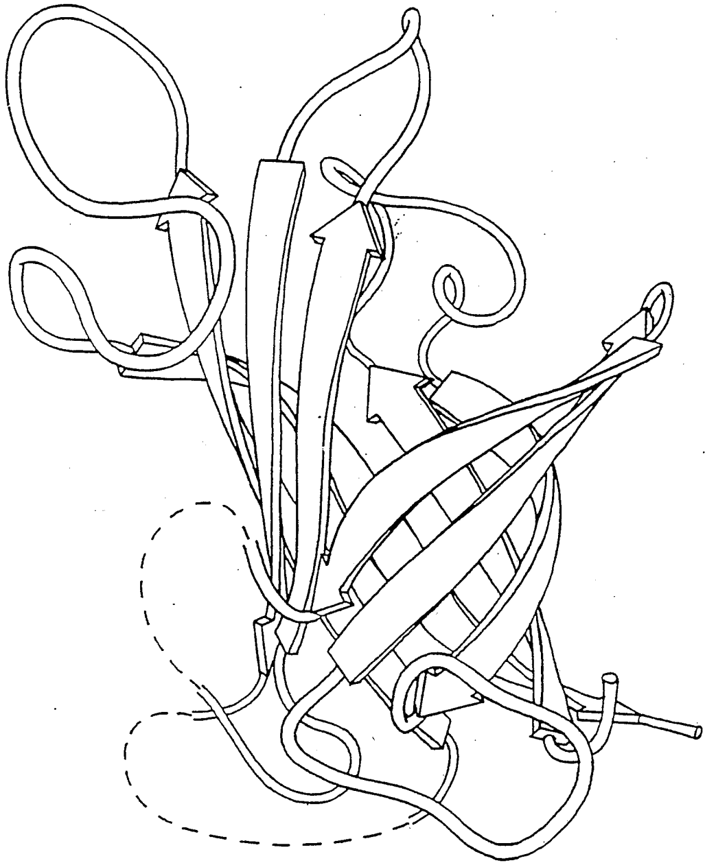
Catalase domain 2
